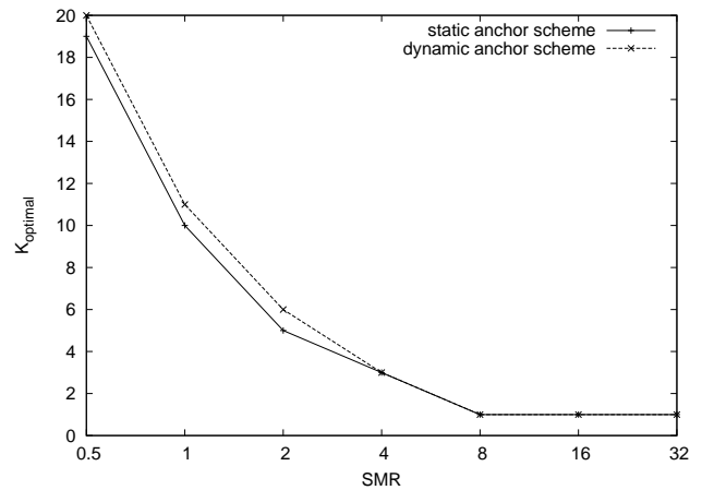
Fig. 8. Optimal K vs. SMR.
